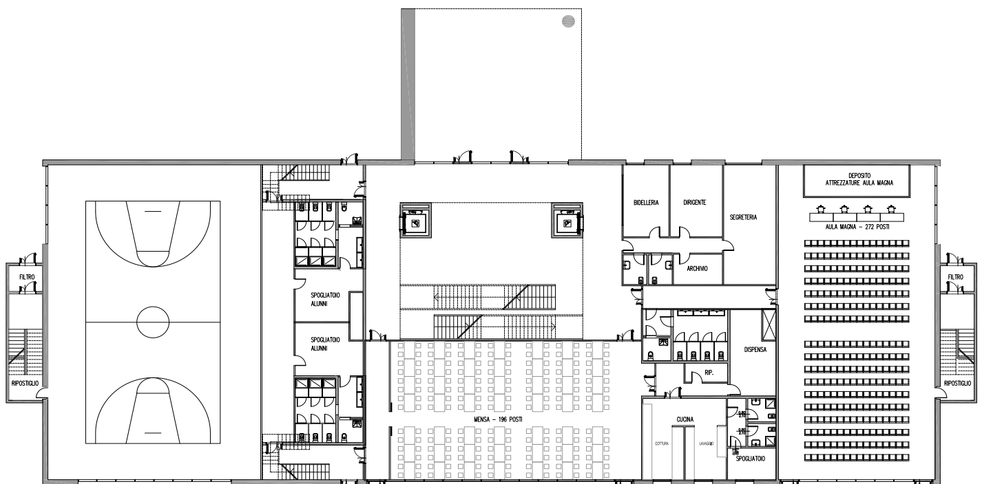
Prospetto da sud-est e pianta piano terra - progetto preliminare nuova scuola media
