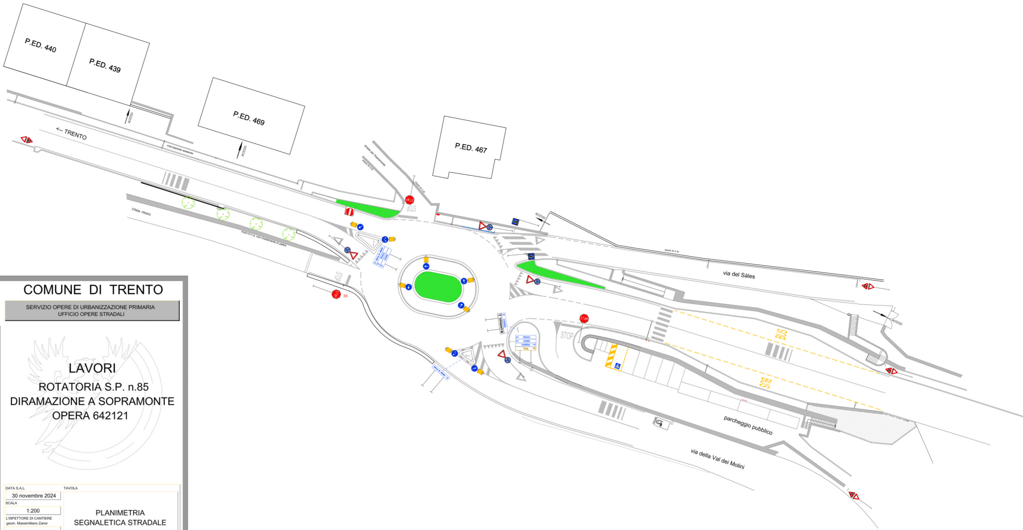
PLANIMETRIA scala 1:200
