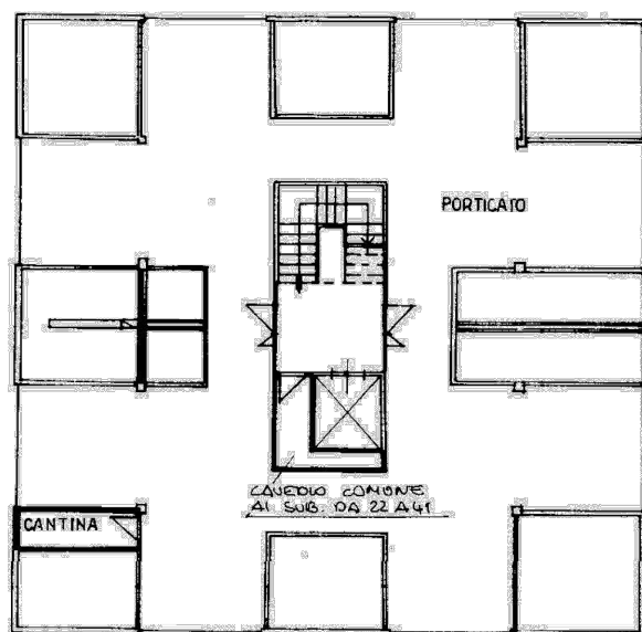
PIANTA PIANO TERRA H=220m
