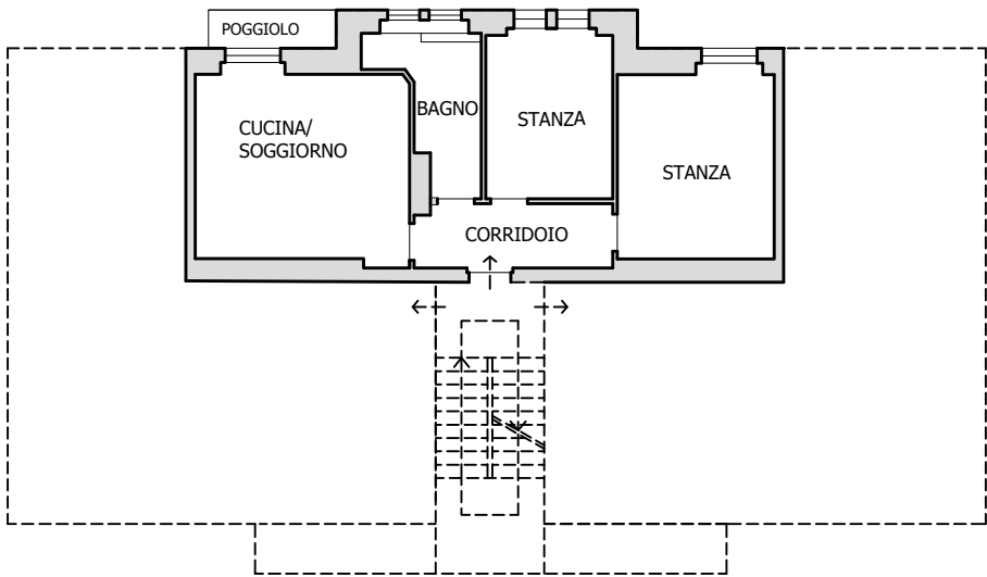
CF 52 - UI 43100645 PIANTA PIANO SECONDO H=2.70m
