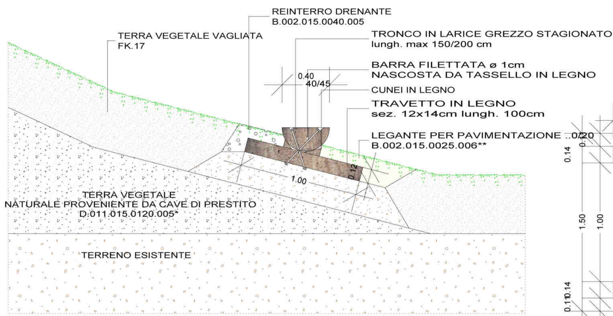
PARTICOLARE SEDUTE RAMPA - Scala 1:20
