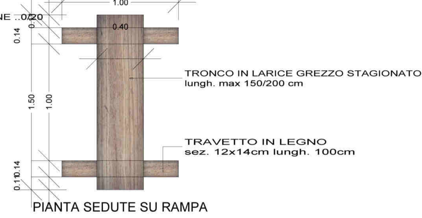
PIANTA SEDUTE SU RAMPA
