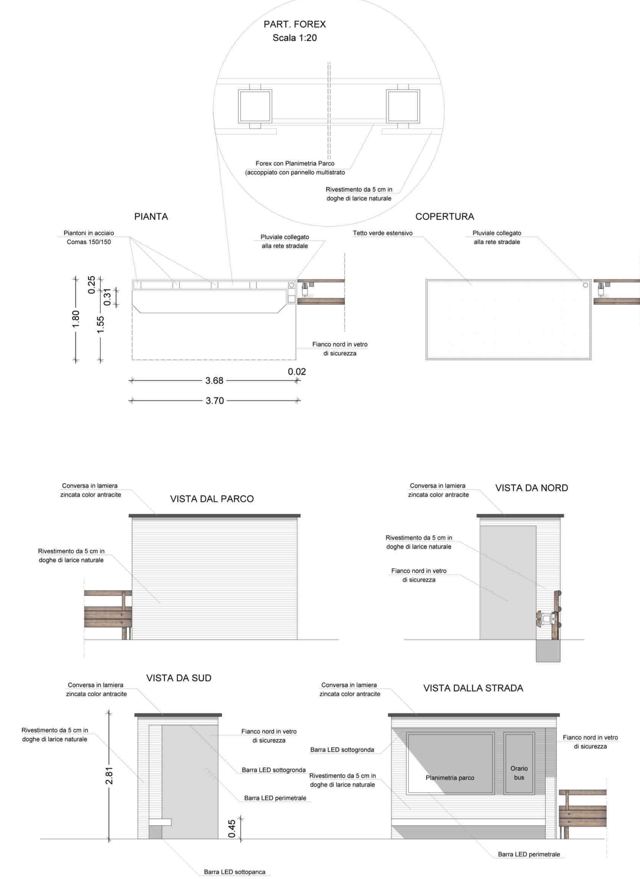
PARTICOLARE PENSILINA AUTOBUS - Scala 1:50
