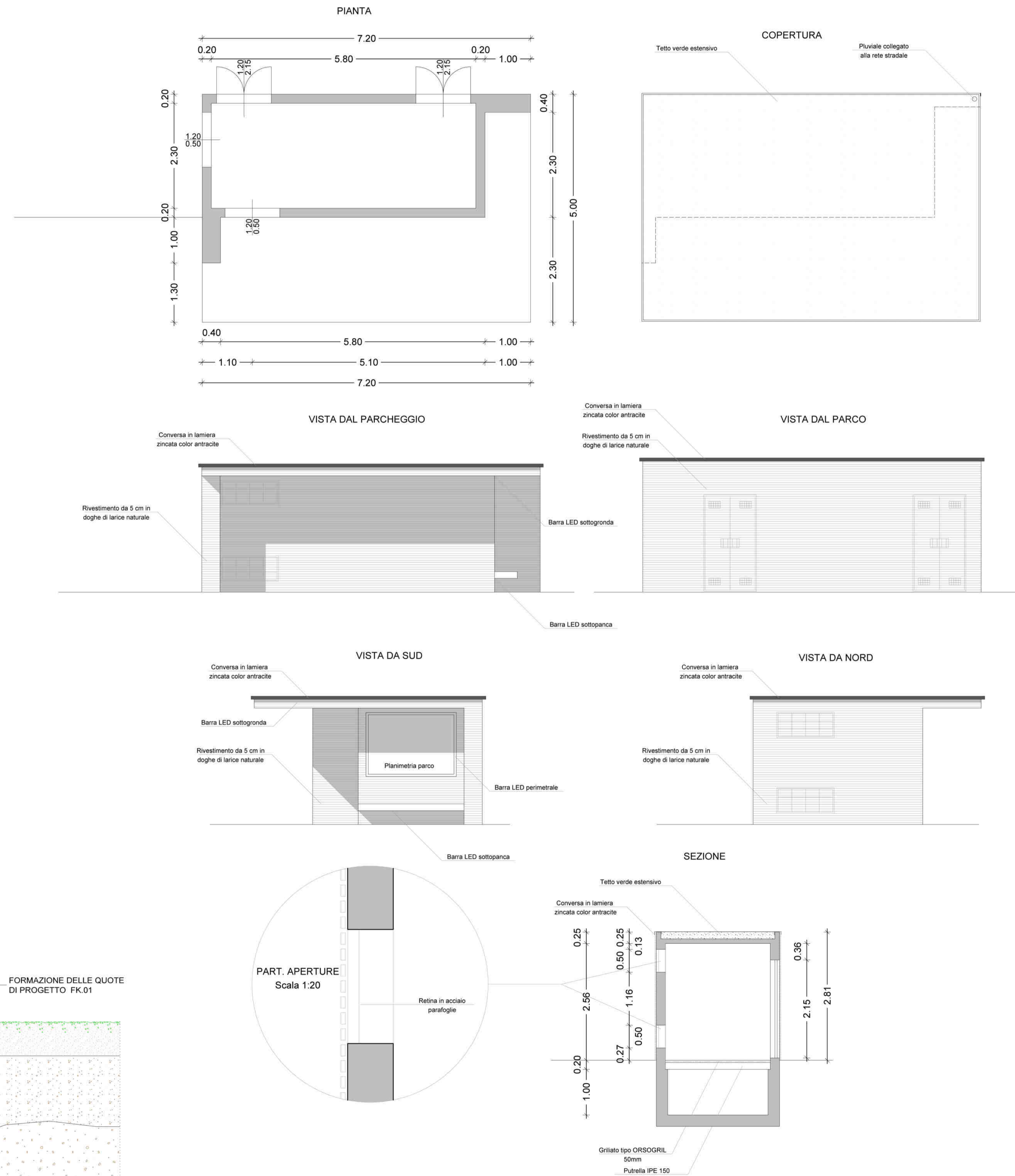
PARTICOLARE CABINA ELETTRICA - Scala 1:50
