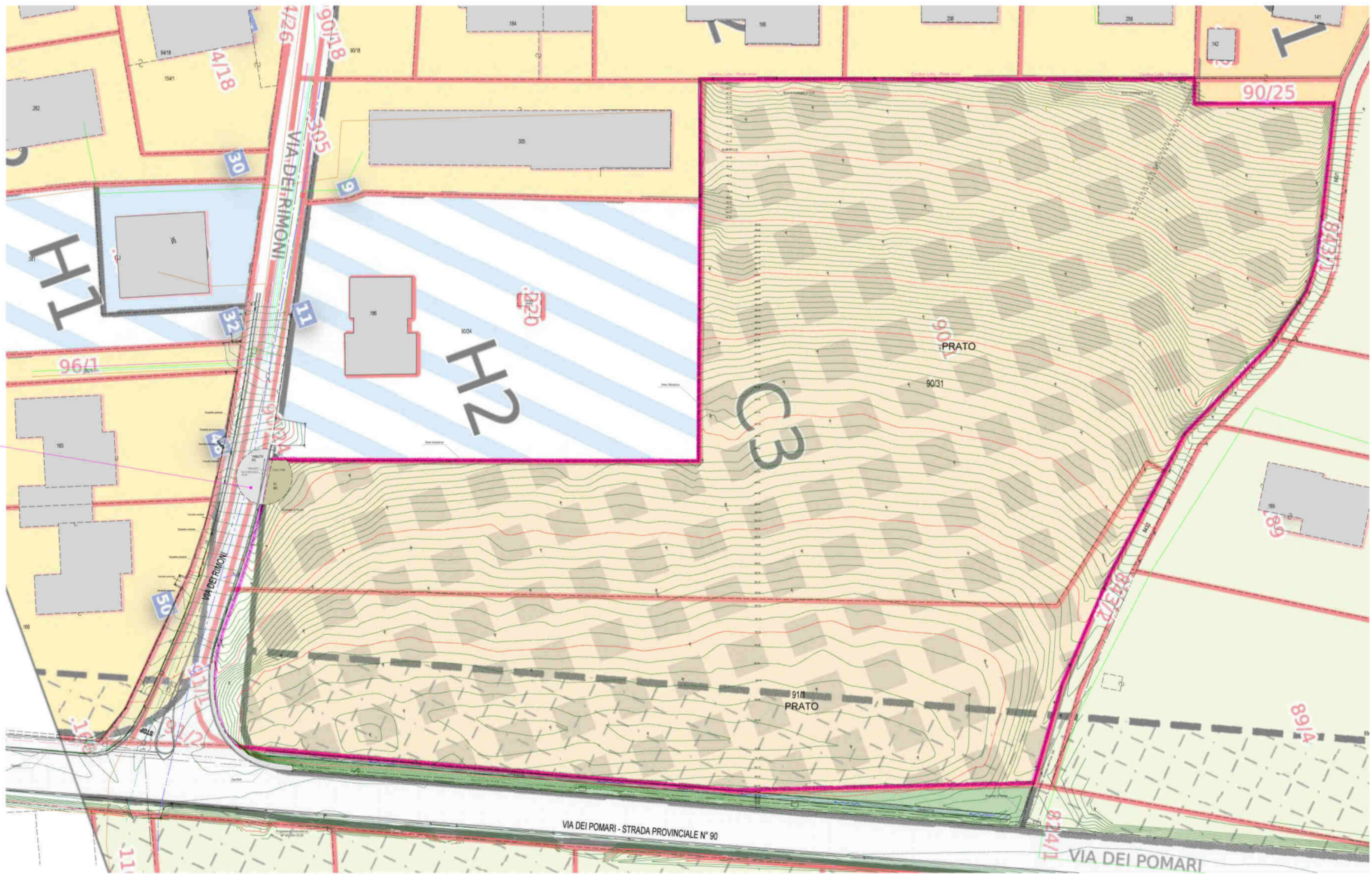
SOVRAPPOSIZIONE RILIEVO STATO ATTUALE CON MAPPA CATASTALE E P.R.G. Scala 1:200
