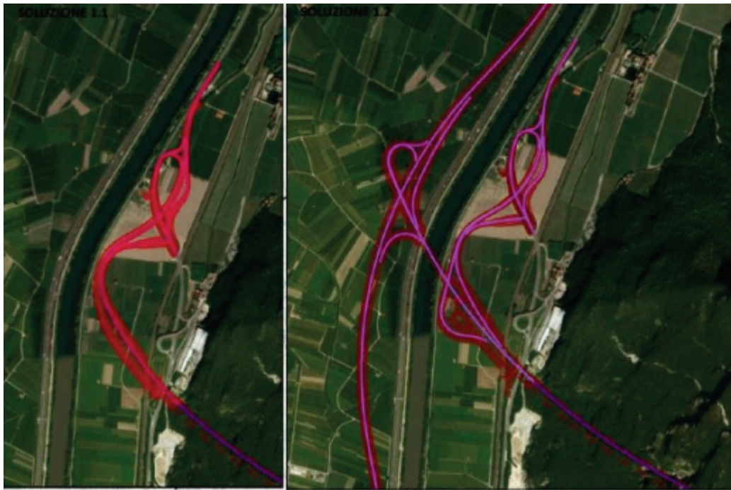
Figura 6.30 Svincolo di Acquaviva - Soluzioni 1.1 e 1.2 su fotopiano
