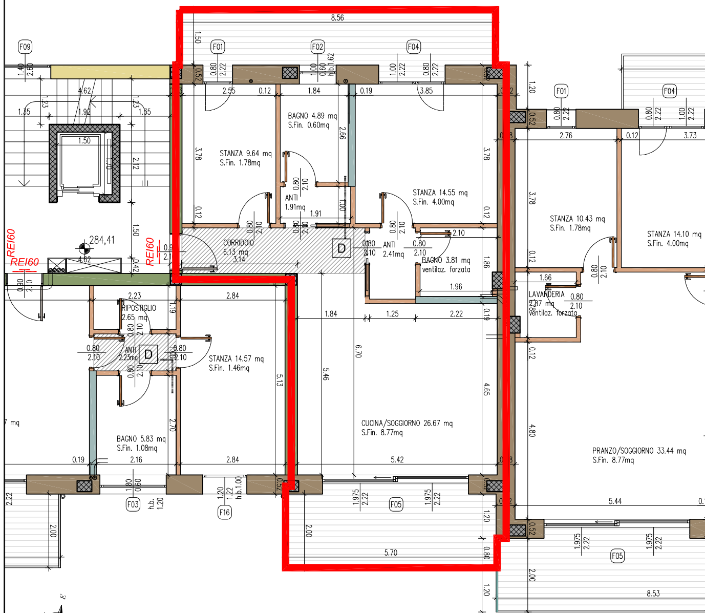
PIANTA APPARTAMENTO E.1.05 scala 1:100
