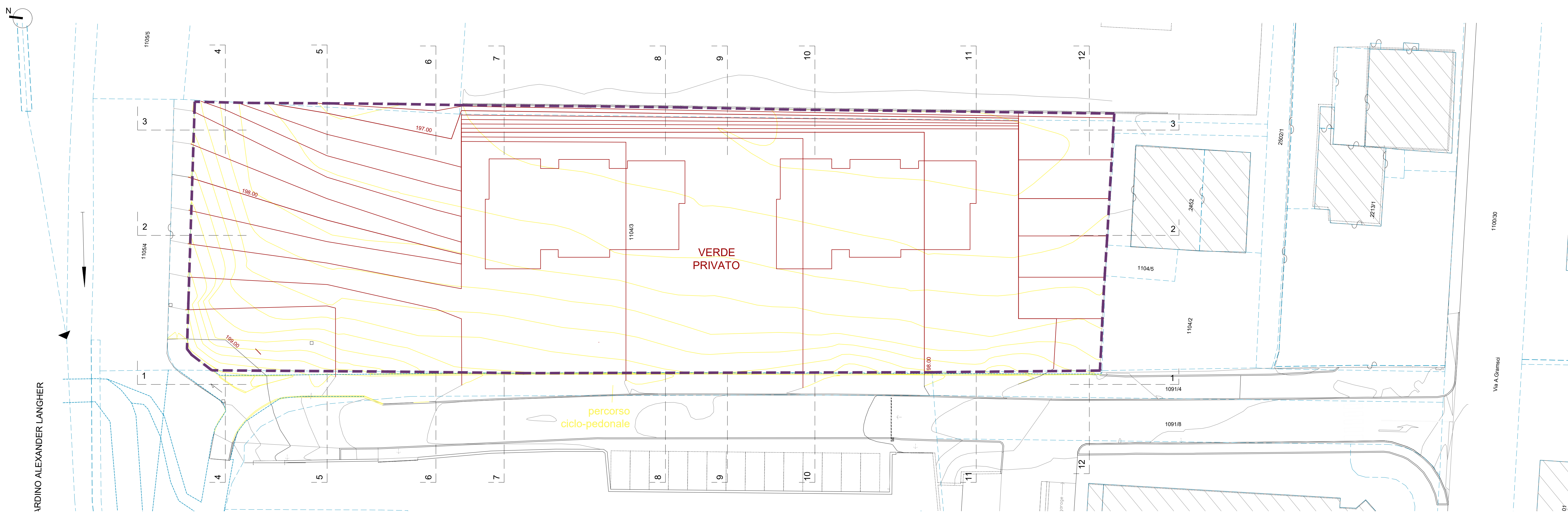
PLANIMETRIA CURVE DI LIVELLO SCALA 1:250
