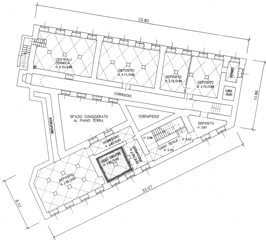
PIANTA PIANO SOTTOSTRADA 1
